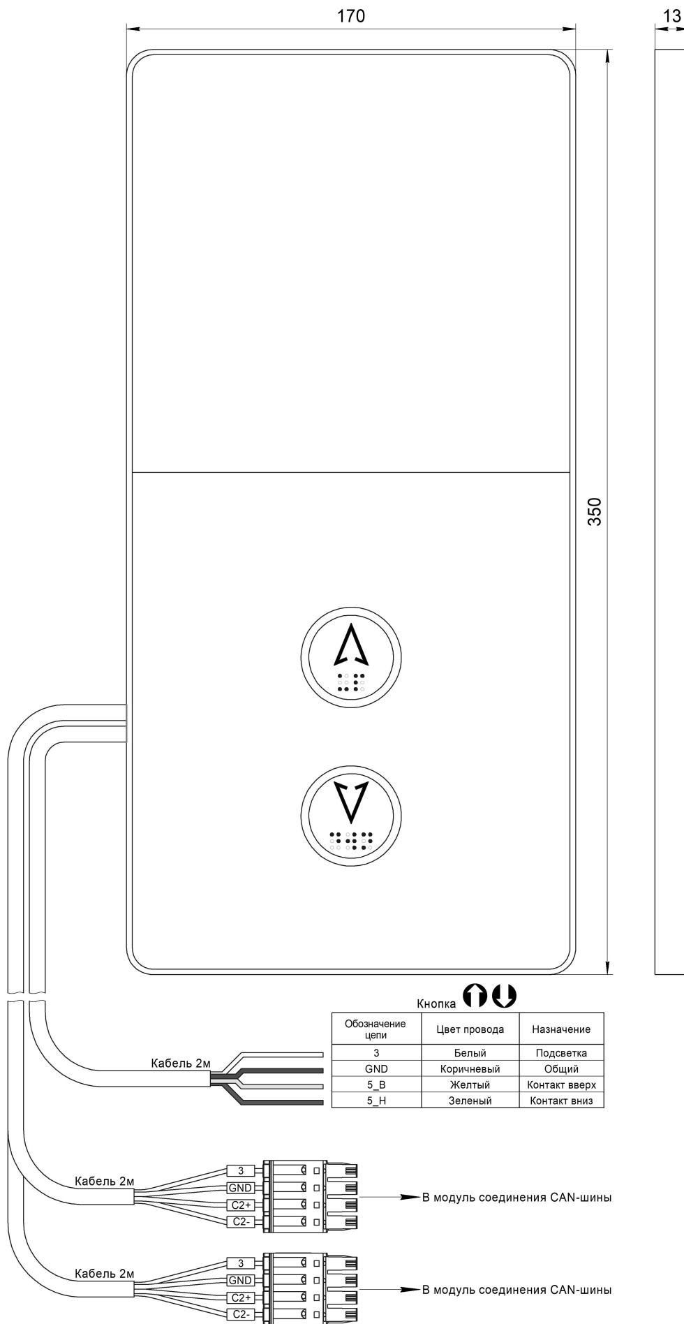
Рис.1 Внешний вид, габаритные и установочные размеры Вызывного поста МАЛАХИТ НШЕК.468381.018
